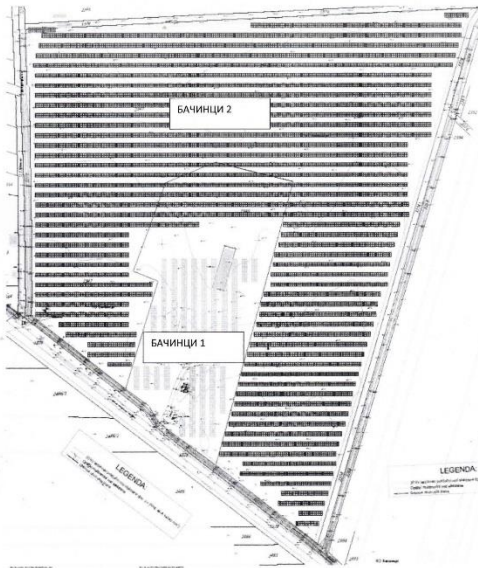
Прелиминарни положај и заузеће парцела СЕ Бачинци 1 и СЕ Бачинци 2
